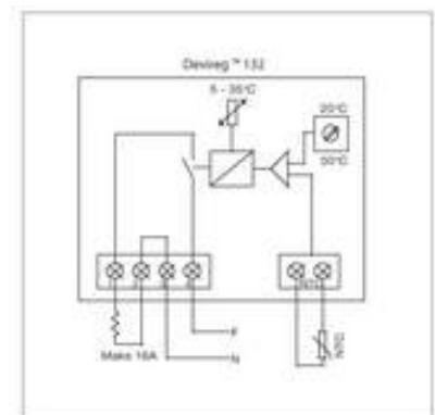
Devireg™ 132
