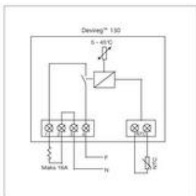
Devireg™ 130
