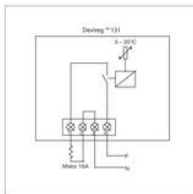
Devireg™ 131
